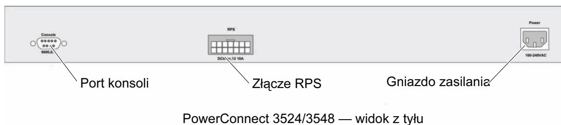
Rysunek 1-3. Złącze zasilania na panelu tylnym
